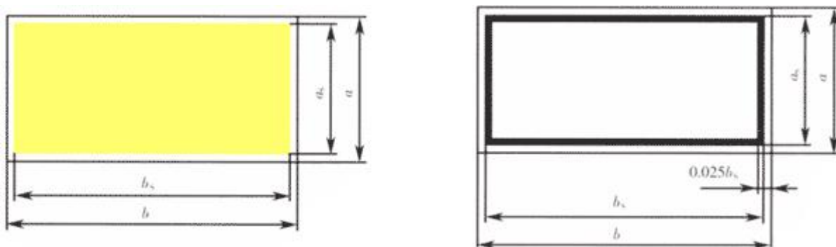
图 A. 5 附加提示标识的基本形式
